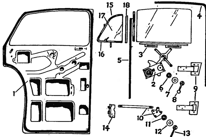
Fig. 7—Rear Door—4-Door Sedans
