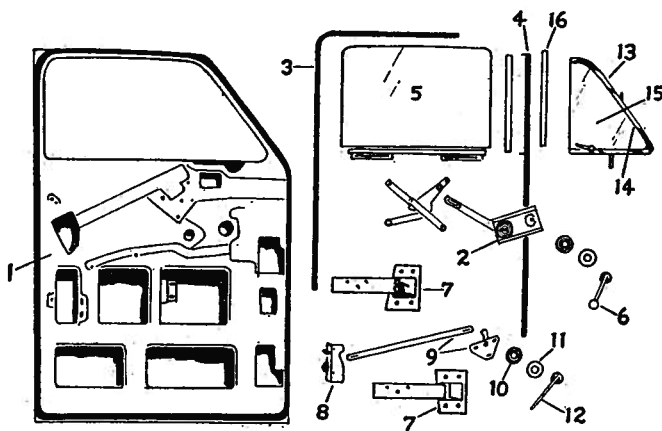
Fig. 6—Front Door—2- & 4-door
