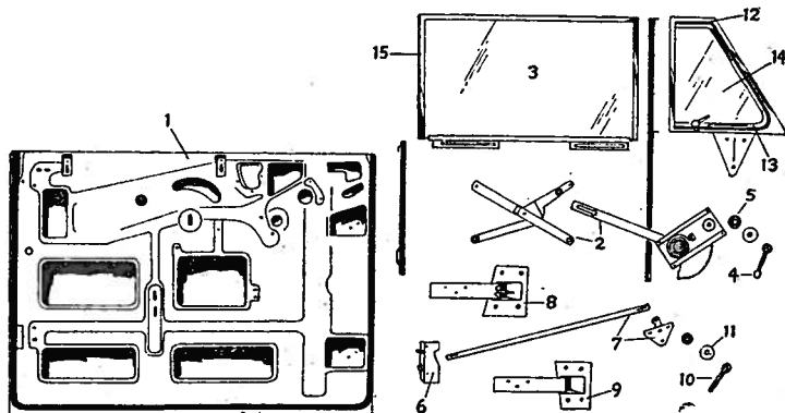
Fig. 13—Door, Convertible
