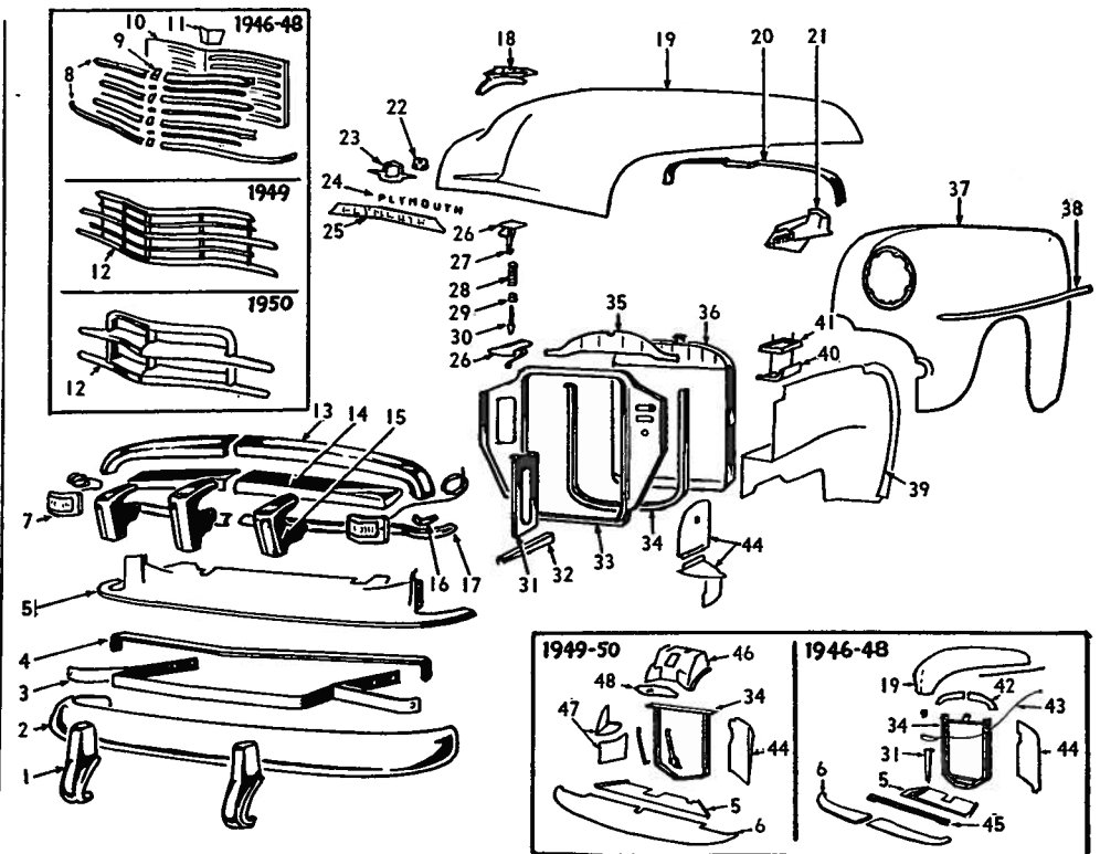
Fig. 1—Sheet Metal—Front End
