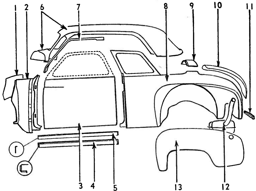
Fig. 2—Body Sheet Metal
