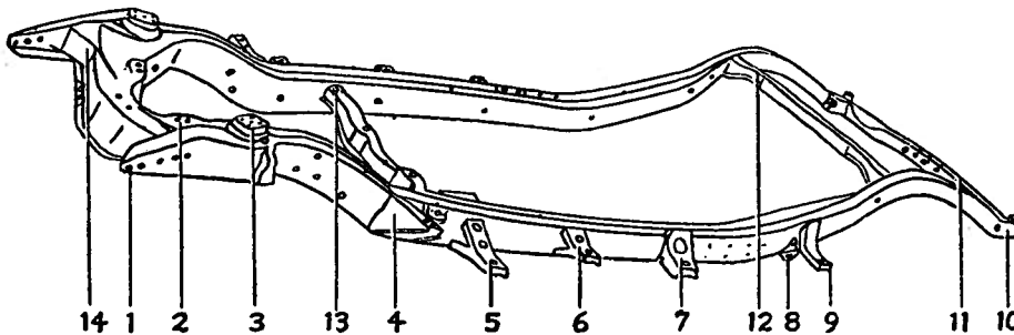
Fig. 15—Frame Assembly
