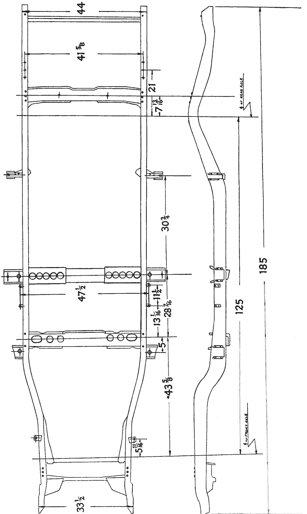
1946-1948 Lincoln Sedan Frame
