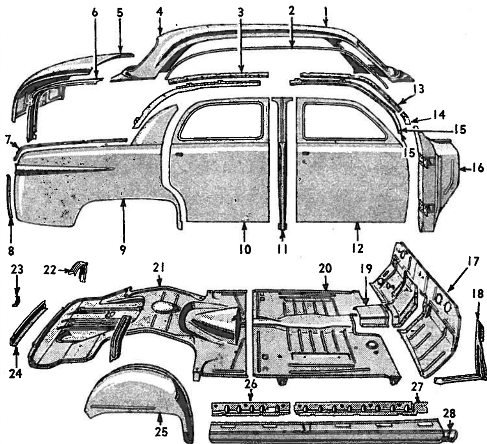
Fig. 4—Body Sheet Metal—Fordor
