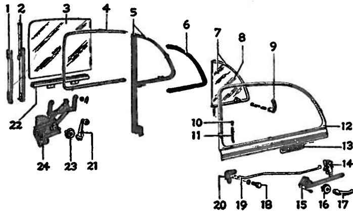
Fig. 7—Rear Door—Body Type 73 Fordor
