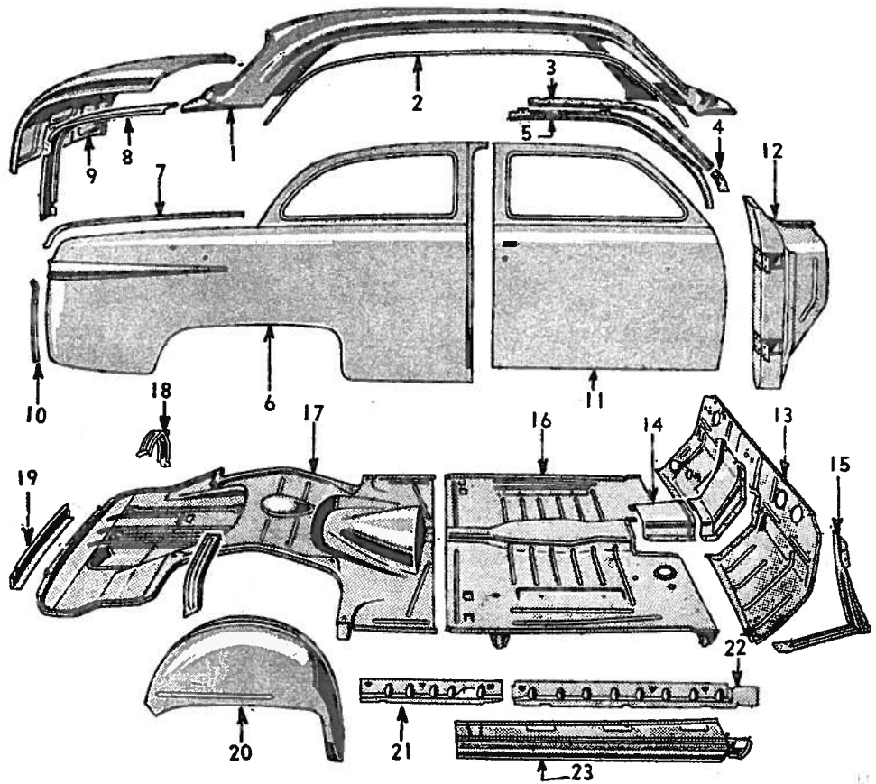
Fig. 10—Sheet Metal—Tudor & Coupes
