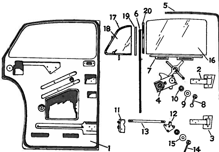
Fig. 5—Rear Door—4-Door Sedans
