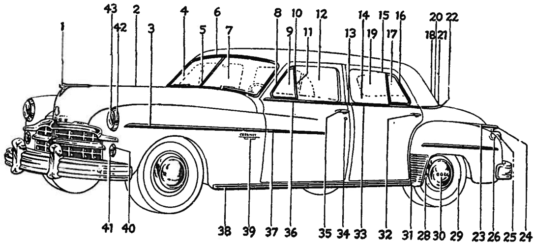
Fig. 2—Body Moldings—4-Door Sedans
