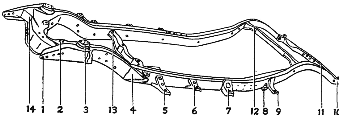
Fig. 13—Frame Assembly
