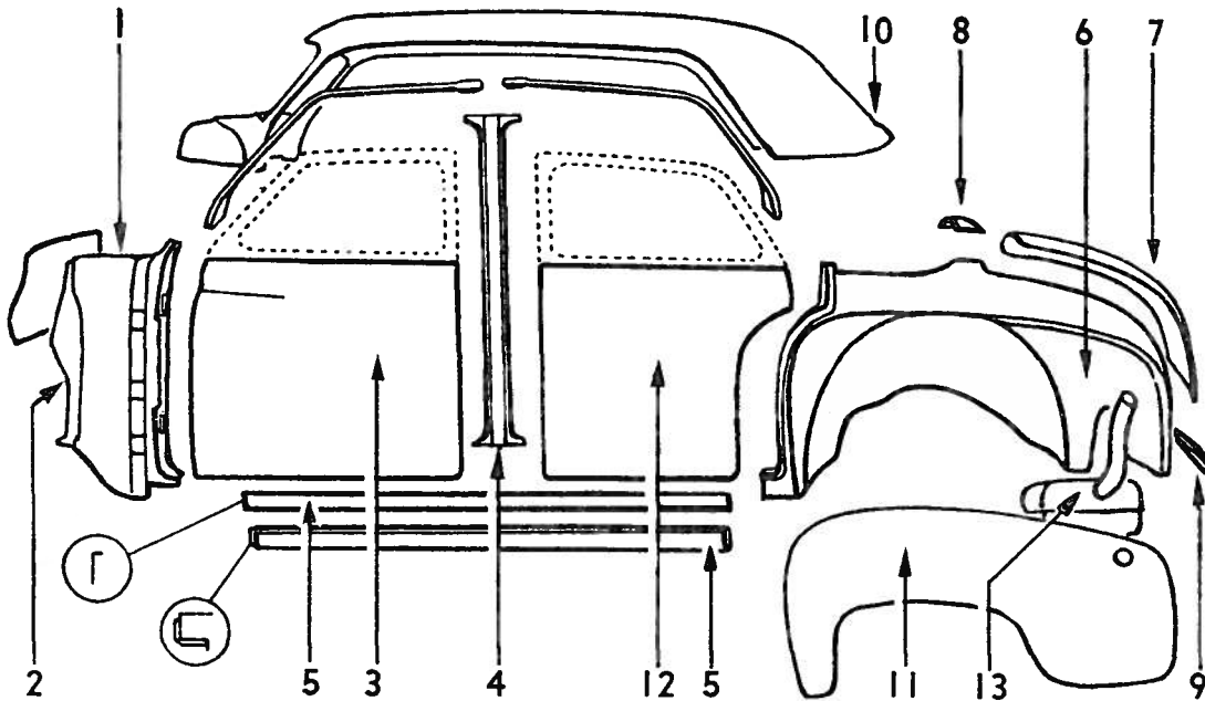
Fig. 3—Body Sheet Metal
