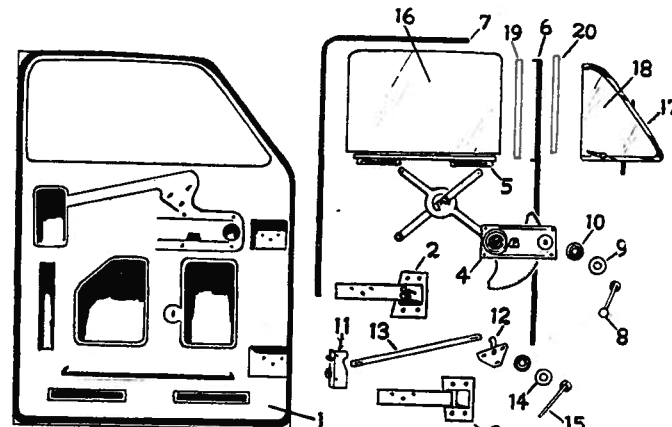
Fig. 4—Front Door Assembly
