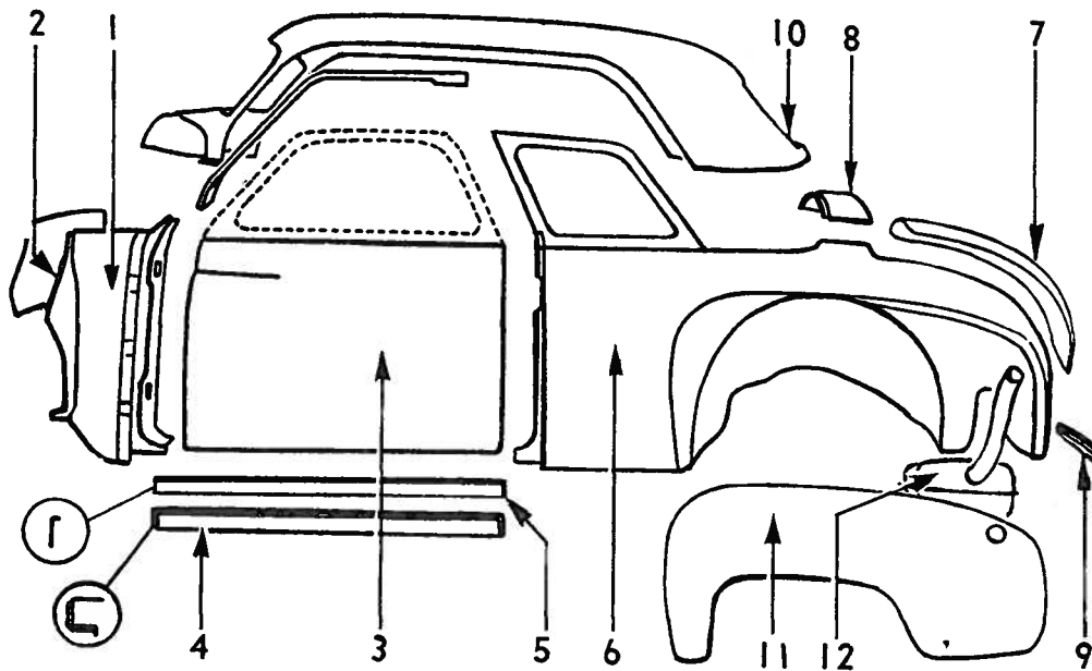
Fig. 7—Body Sheet Metal
