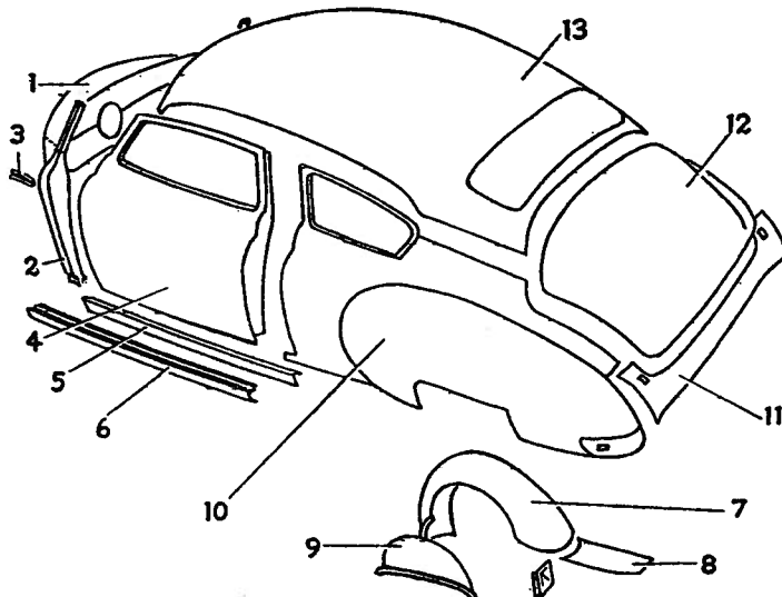
Fig. 4—Body sheet metal
