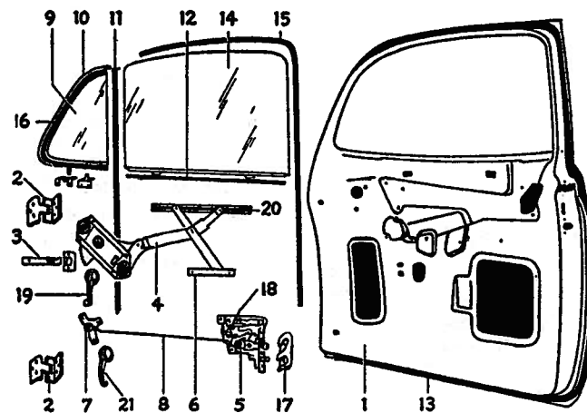
Fig. 15—Front Door—Typical of all 2-4 Door
