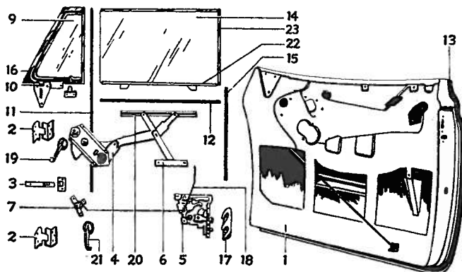
Fig. 14—Front Door (Left Side Part Numbers Shown) Cabriolet & Bel Air
