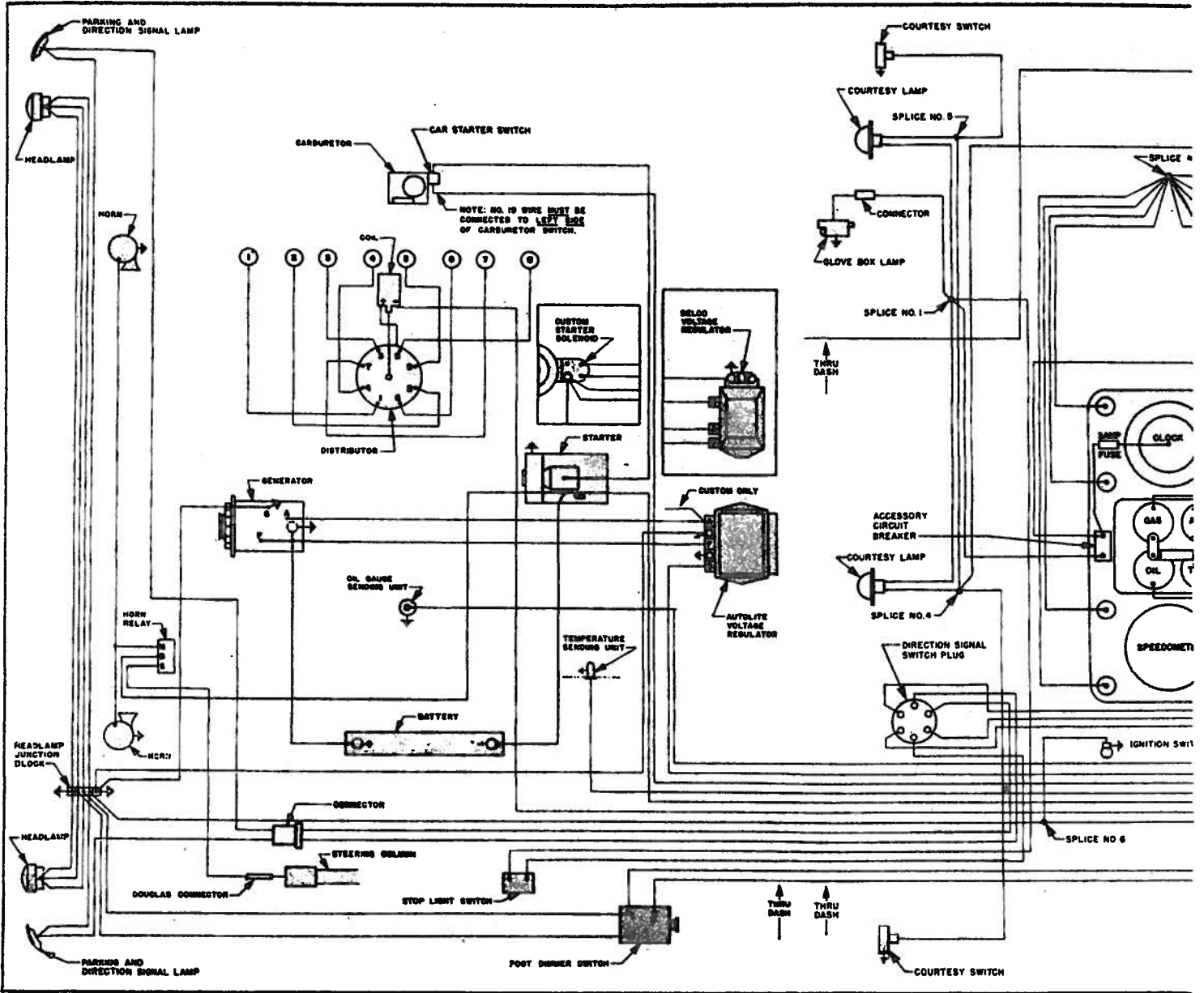
Wiring Diagram—
