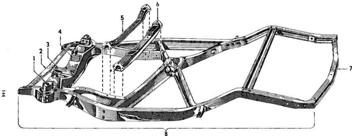
Fig. 9—Frame Assembly
