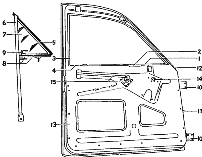
Fig. 5—Front Door Assembly
