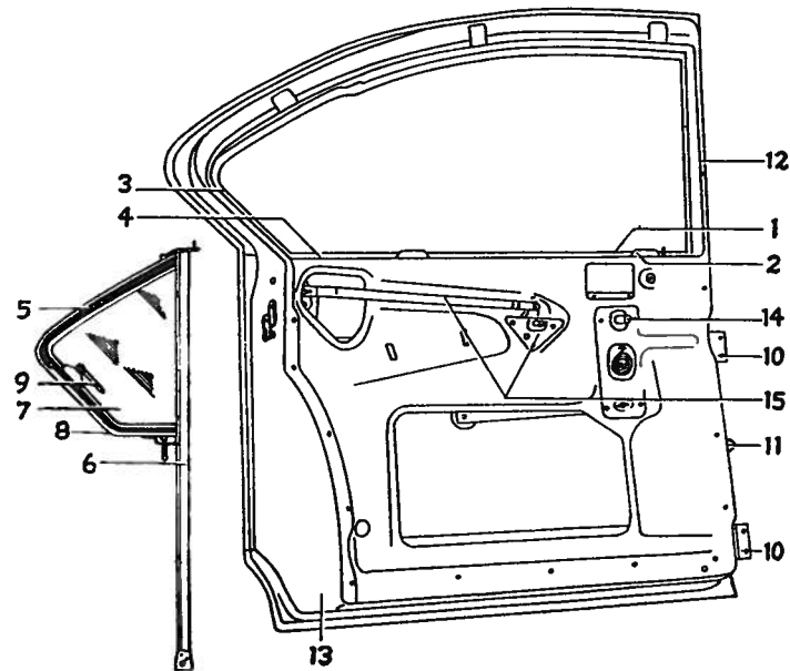
Fig. 6—Rear Door Assembly
